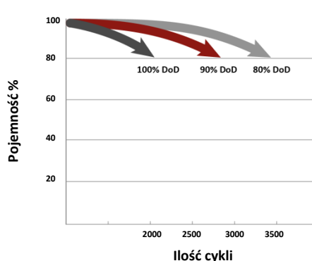
Żywotność cykliczna w funkcji głębokości rozładowania DoD:
